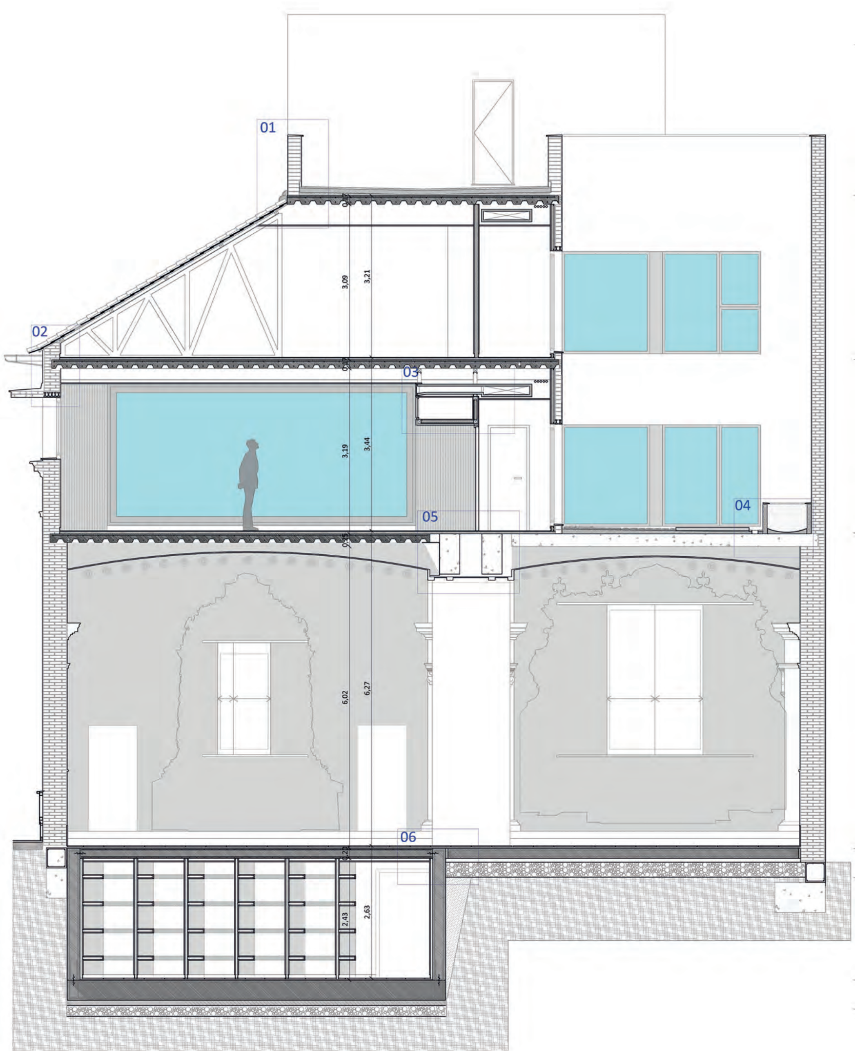
Sección 1: Alzado
